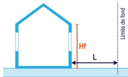
Façades sans baie : L \geq H_f et L \geq 8m
