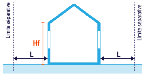
Façades avec baie : L \geq H_f et L \geq 5m
