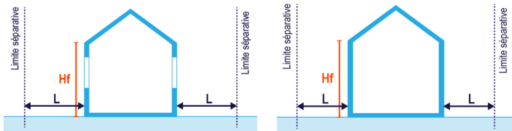
Façades sans baie : L \geq H_f/2 et L \geq 3m
