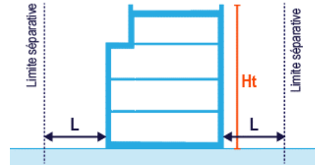
Façades sans baie : L \geq (Ht/2)-3m et L \geq 3m
