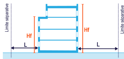
Façades avec baie : L \geq (Hf/2)-3m et L \geq 5m
