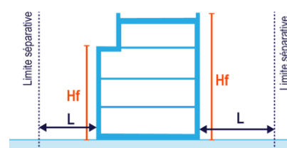
Façades sans baie : L \geq (Hf/2)-3m et L \geq 3m
