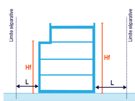
Façades sans baie : L \geq (Hf/2)-3m et L \geq 2m
